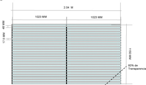
EJEMPLO DE INSTALACION DE PANTALLA CON 48 BARRAS
